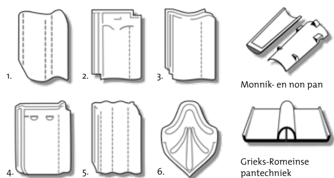
1. oud-Hollandse pan, 2. verbeterde oud-Hollandse pan, 3. opnieuw verbeterde oud-Hollandse pan, 4. Tuile-du-Nord, 5. gegolfde Friese pan, 6. Oegstgeester pan.
