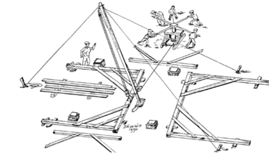
Het opzetten van een vierkantsconstructie met een kaapstander.
