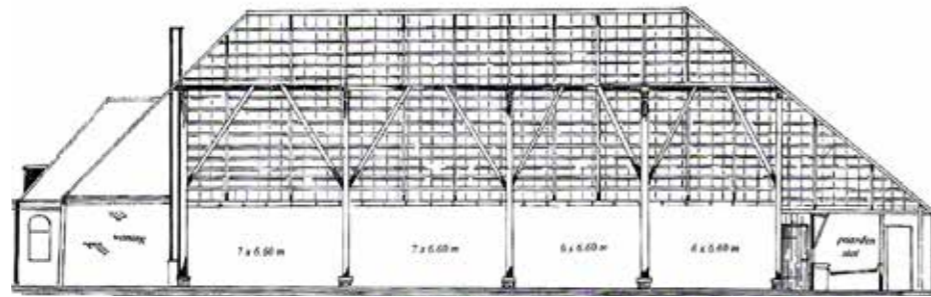
Dwarsdoorsnede van de schuur van de hoeve 'Zeeland', Anna Paulowna (1901).
